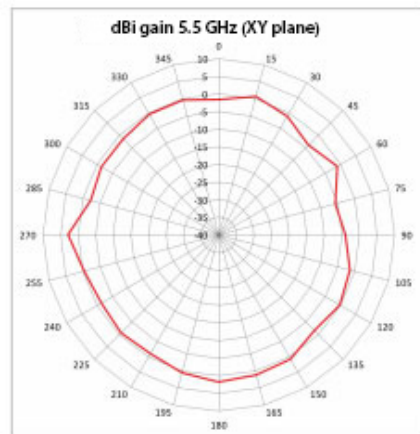
5 GHz Antenna
